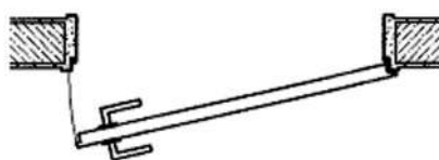
Vue du côté ferrage Ferrage à droite = DIN Droite
